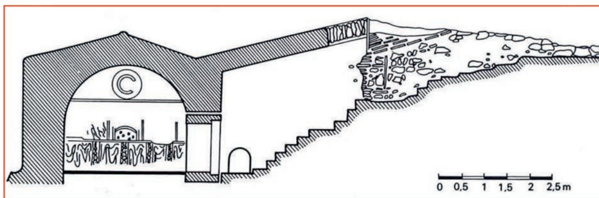
План и надлъжен разрез на „Хисарската гробница“, проучена от Христо Джамбов през 1957 г.
